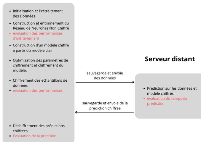
Figure 6 - Schéma d'utilisation de la librairie HElayers
